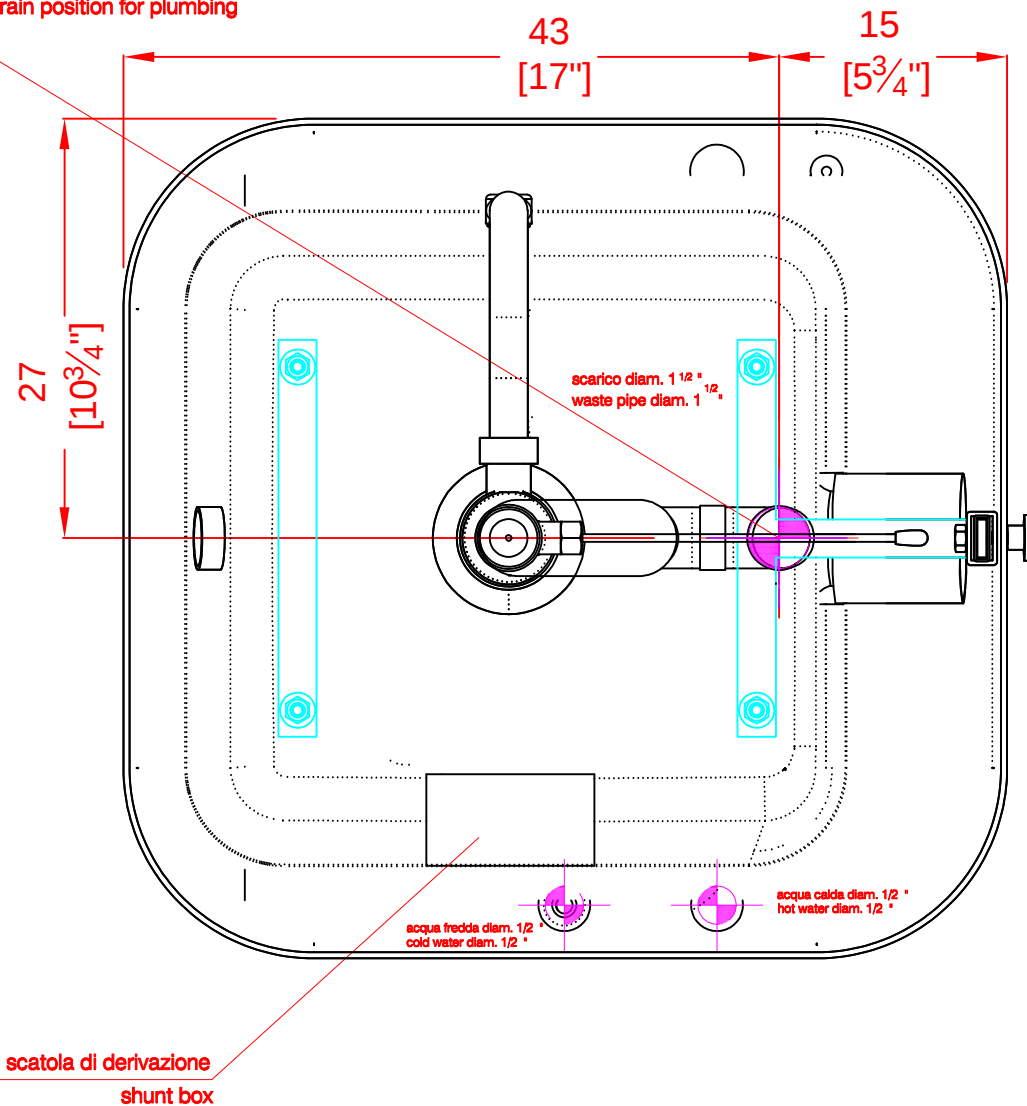
posizione scarico acqua a pavimento drain position for plumbing
